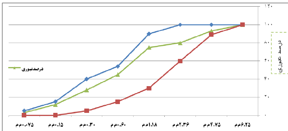
شکل ۲- منحنی دانه بندی ماسه مصرفی
