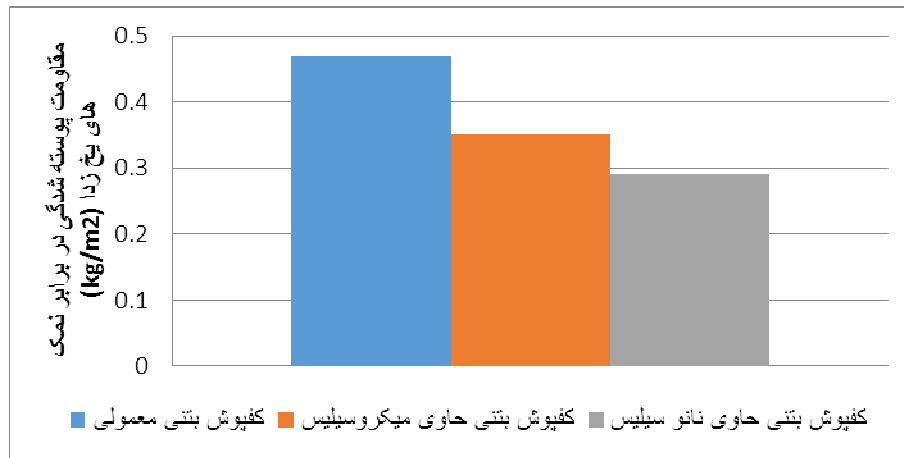
شکل ۹- نتایج آزمون مقاومت پوسته شدگی در برابر نمک های یخ زدا کفپوش های بتنی ترافیکی
