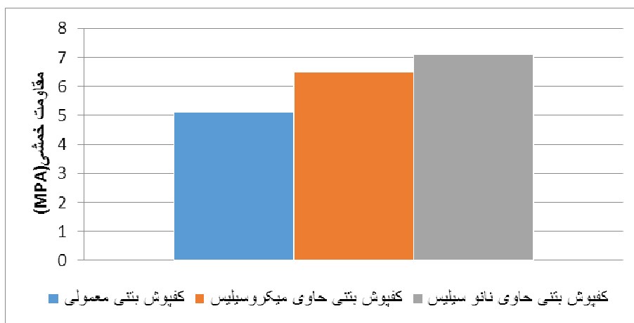
شکل ۵- نتایج آزمون مقاومت خمشی کفپوش های بتنی ترافیکی
