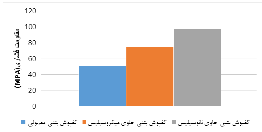
شکل ۲- نتایج آزمون مقاومت فشاری کفپوش‌های بتنی ترافیکی
