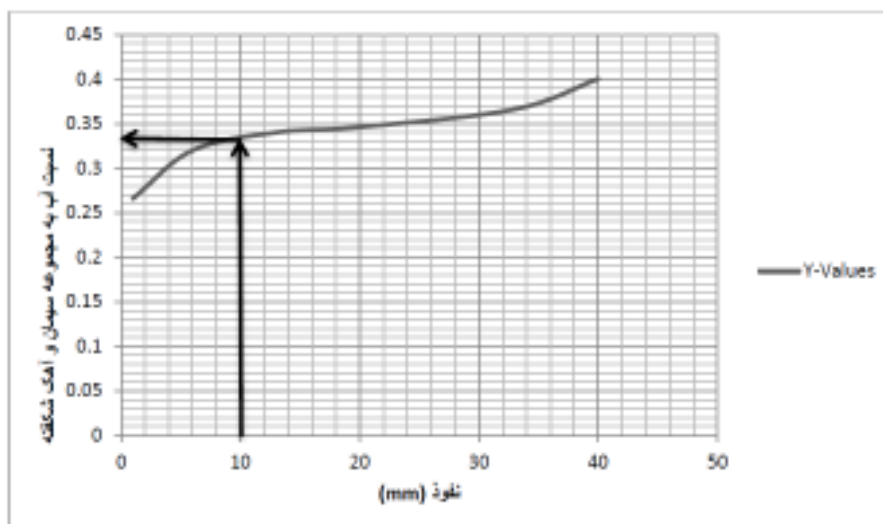
شکل ۲- منحنی نسبت آب به مواد سیمانی و میزان نفوذ سوزن ویکات بر حسب میلی متر
