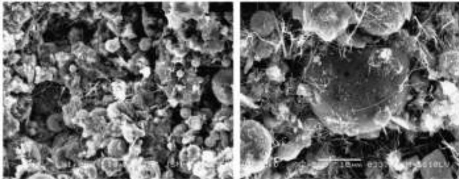
شکل ۱- نمایش میکروسکوپی وضعیت توپرشدگی فضاهای خالی و کاهش نفوذپذیری ملات های آهکی خاکستر دار
