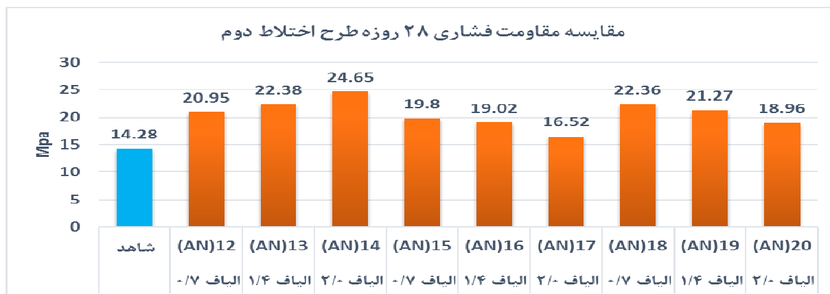
نمودار ۶- نمودار مقاومت فشاری ۲۸ روزه طرح اختلاط دوم با نسبت آب به سیمان ۰/۵
