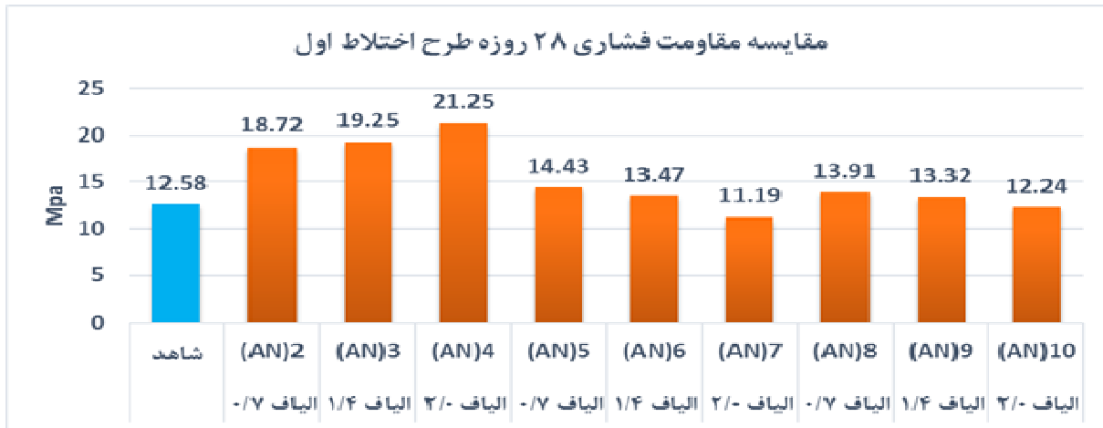
نمودار ۴- نمودار مقاومت فشاری ۲۸ روزه طرح اختلاط اول با نسبت آب به سیمان ۰/۵۵
