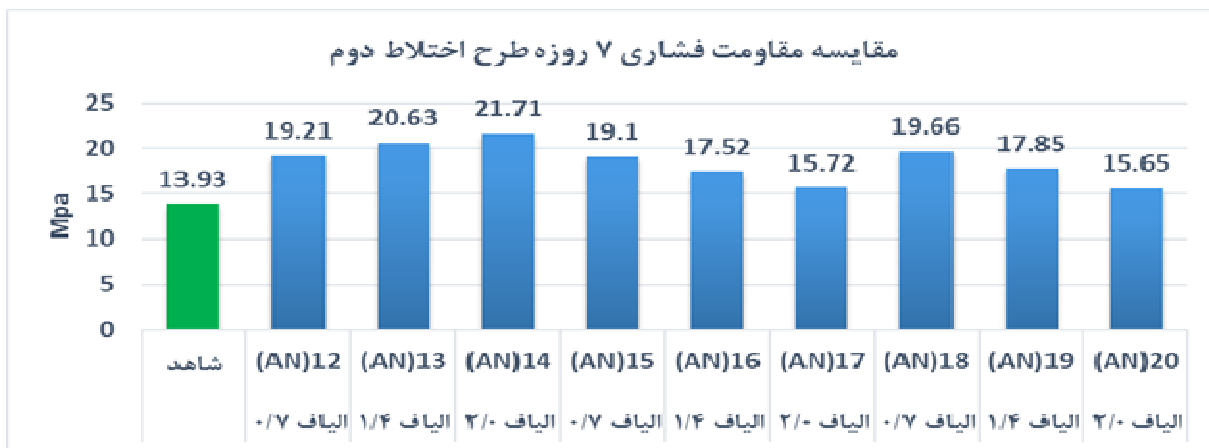
نمودار ۵- نمودار مقاومت فشاری ۷ روزه طرح اختلاط دوم با نسبت آب به سیمان ۰/۵
