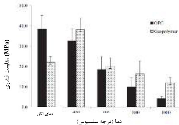
شکل ۱۰- نمودار مقاومت فشاری نمونه‌های بتن ژئوپلیمر (Geopolymer) و بتن معمولی (OPC) در دماهای بالا و سپس خنک‌سازی در هوا [12]
