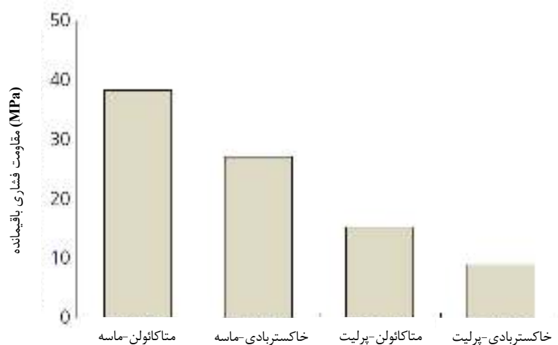
شکل ۶- نمودار مقاومت فشاری باقیمانده پس از عبور از دمای ۶۰۰ درجه سلسیوس [21]
