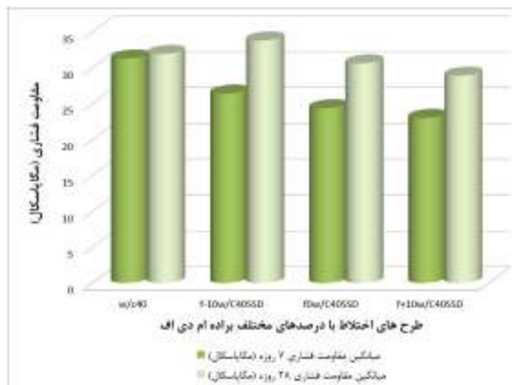
شکل ۳- مقاومت فشاری طرح های با نسبت آب به سیمان ۰/۴ و استفاده از فیبر اشباع
