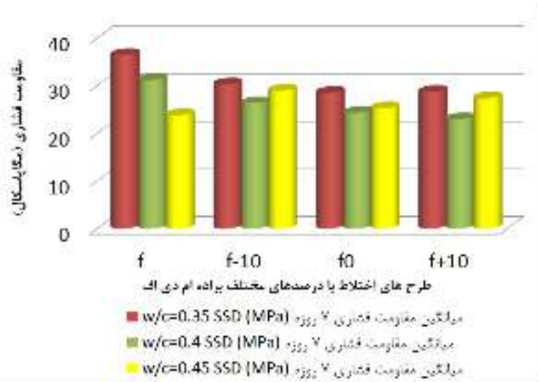
شکل ۷- مقایسه ی مقاومت های فشاری ۷ روزه در حالت فیلر اشباع شده با نسبت آب به سیمان های مختلف
