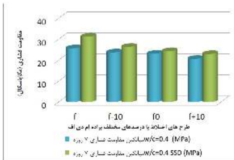
شکل ۵- مقایسه ی مقاومت های فشاری ۷ روزه در نسبت آب به سیمن های مختلف ۰،۴ در حالت خشک و اشباع فیلر
