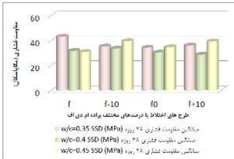
شکل ۸- مقایسه ی مقاومت های فشاری ۲۸ روزه در حالت فیلر اشباع شده با نسبت آب به سیمان های مختلف
