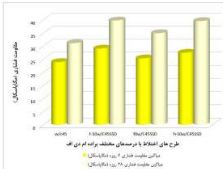
شکل ۴- مقاومت فشاری طرح های با نسبت آب به سیمن ۰/۴۵ و استفاده از فیلر اشباع
