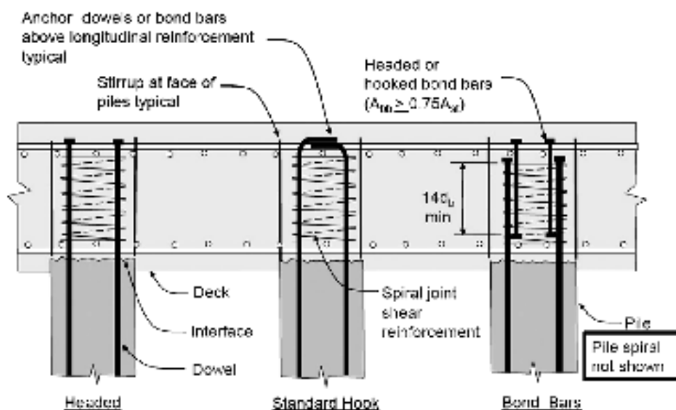
شکل ۴- جزئیات اتصال ترک خورده سرشمع شمع بتنی [۱۷]
